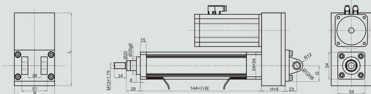
DMB10尾座铰接安装形式-RC
