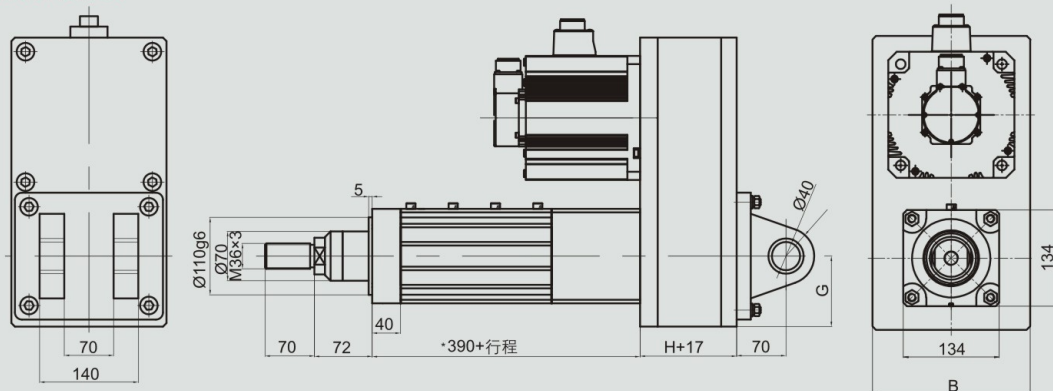
DMB50尾座铰接安装形式-RC
