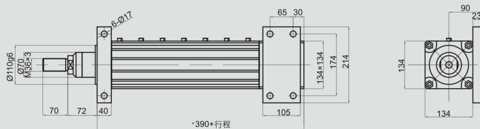
DMB50侧面法兰安装形式-SF
