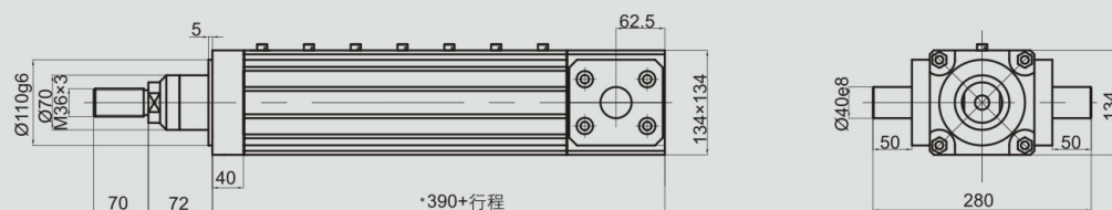
DMB50耳轴安装形式-ST
